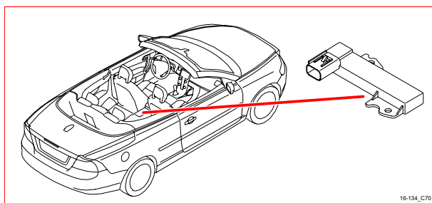
16/134 後車廂車門鎖天線 2，C70
