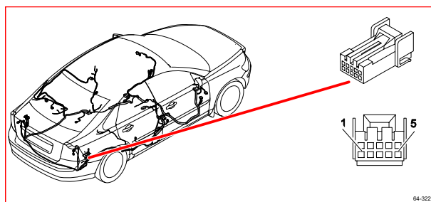
64/322 接頭
