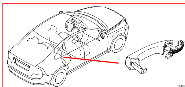
16/131 天線，右後車門鎖
