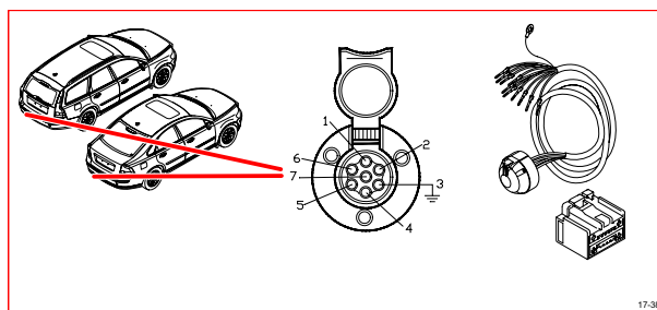
17/38 拖車鉤電線束 7 腳插座
