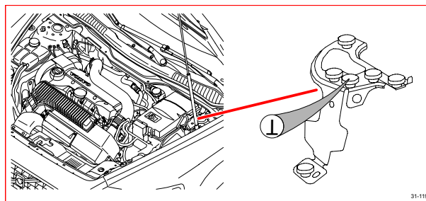
31/119 接地，左側麥弗森懸架
