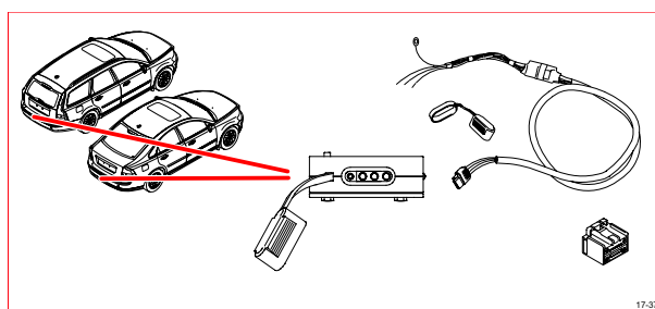
17/37 拖車鉤電線束 4 腳插座
