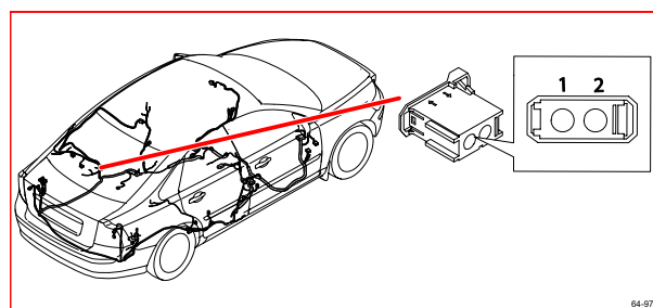
64/979 接頭
