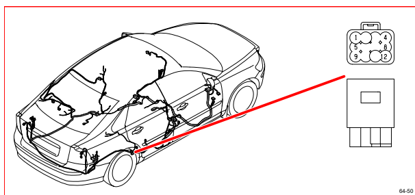
64/50 接頭
