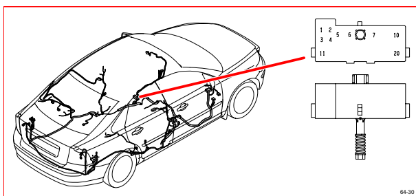
64/30 接頭
