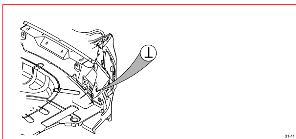
31/11 接地，左後側
