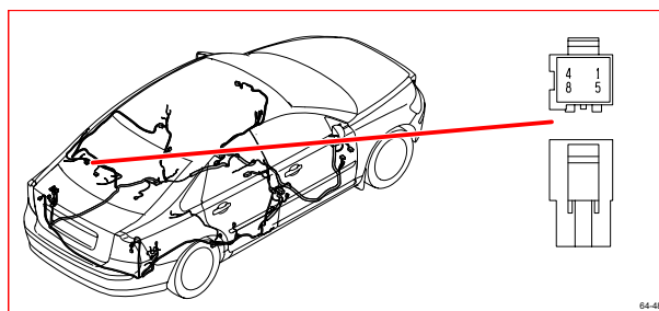
64/48 接頭，S40/V50
