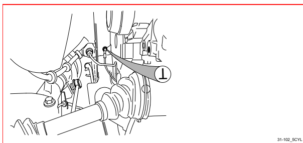
31/102 接地，前橫樑構件，5 缸
