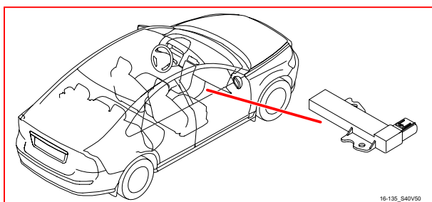
16/135 後車廂車門鎖天線 3，S40/V50
