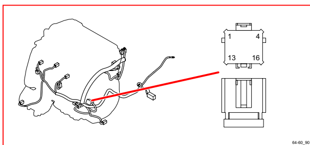
64/60 接頭
