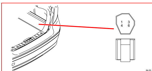
64/53 接頭
