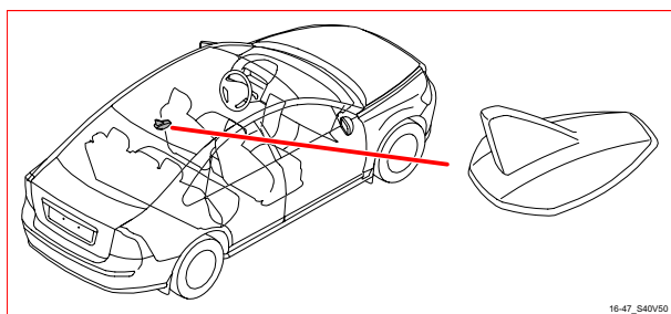
16/47 天線 GSM/GPS/RDAR , S40/V50
