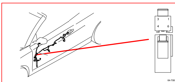
64/708 接頭
