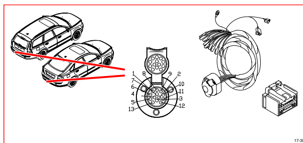
17/39 拖車鉤電線束 13 腳插座
