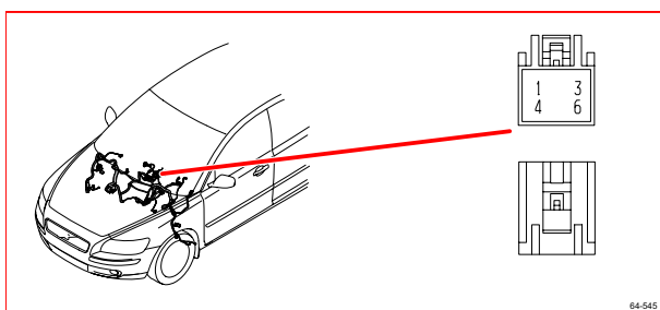
64/545 接頭
