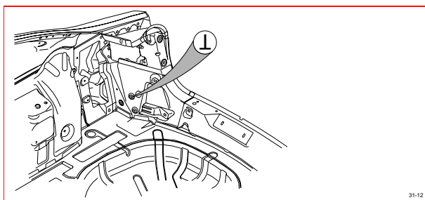
31/12 接地，右後側
